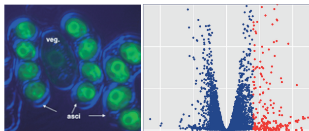
図3. 分裂酵母の胞子（左）と発現遺伝子の比較解析（右）
