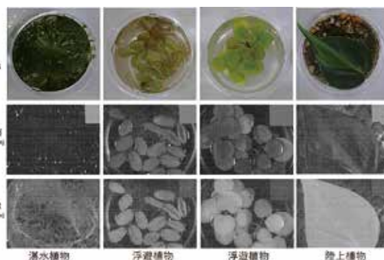
図2. 植物の形態と可視光・赤外線反射特性 潜水性植物は近赤外線(NIR)の反射が小さいが、浮遊植物では陸上植物と同等の強い反射光の観測が期待できる。
